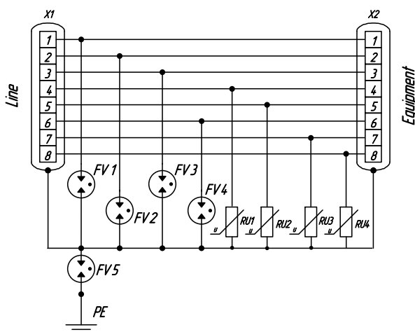
Рисунок 2. Функциональная схема устройства Commeng FEP-m f/f
